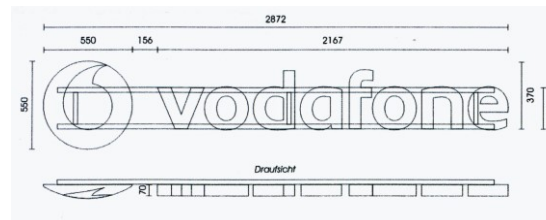
Einzelbuchstaben auf metallischer Unterkonstruktion
