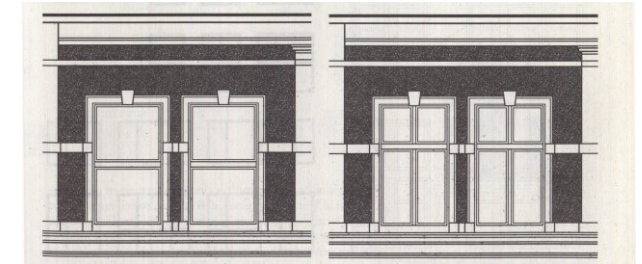
Fensterkämpfer und Kämpfergesims bilden an späthistorischen Bauten eine durchgehende Linie (Darstellung 2), die nicht wie in Darstellung 1 missachtet werden darf
