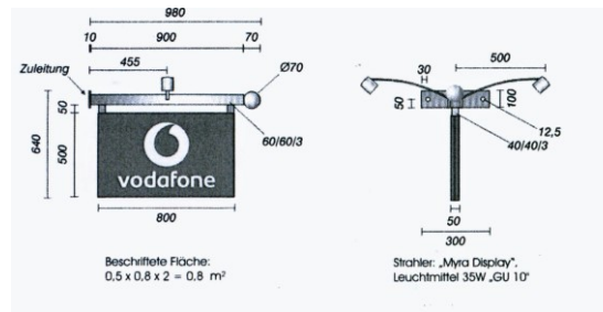
auskragende Werbeanlage
