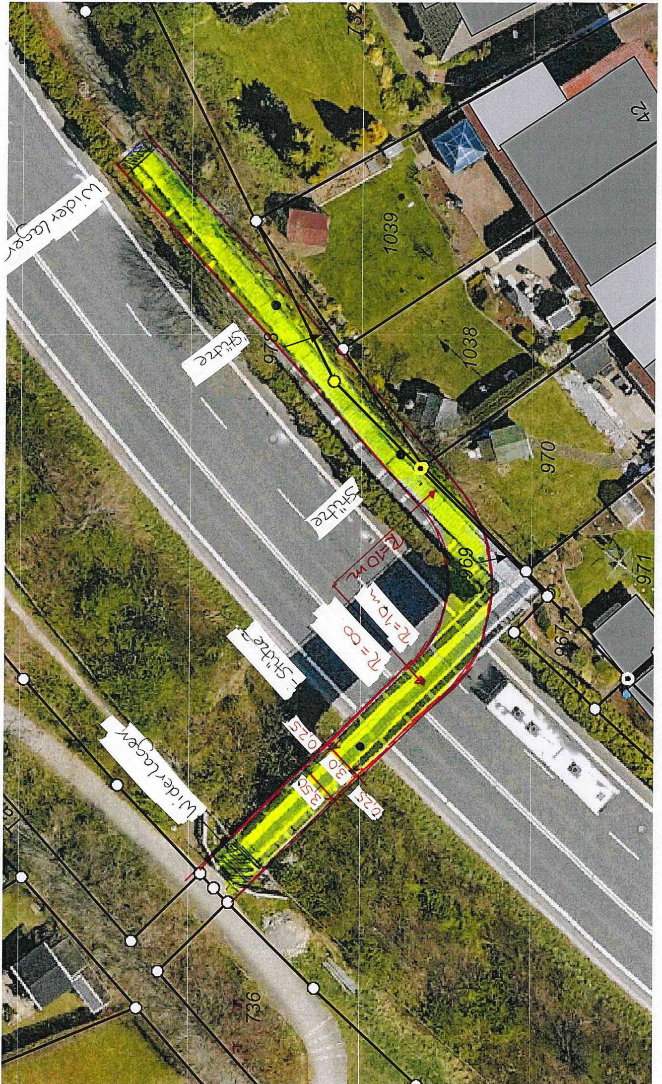
Entwurf Brücke Läsénbacher Landsh. M \approx 1:280
