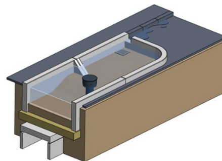
Tiefbeet-Bodenfilter Innodrain
